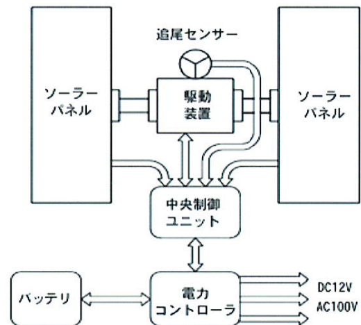
〈ブロック図〉
