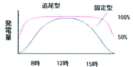
〈追尾型と固定型の発電量の比較〉
